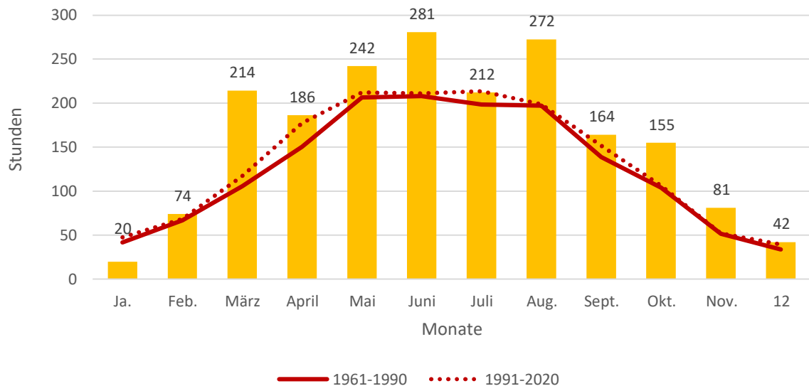
Abbildung XI.2 Durchschnittliche monatliche Sonnenstunden 2022 und langjähriges Mittel 1961 bis 1990
