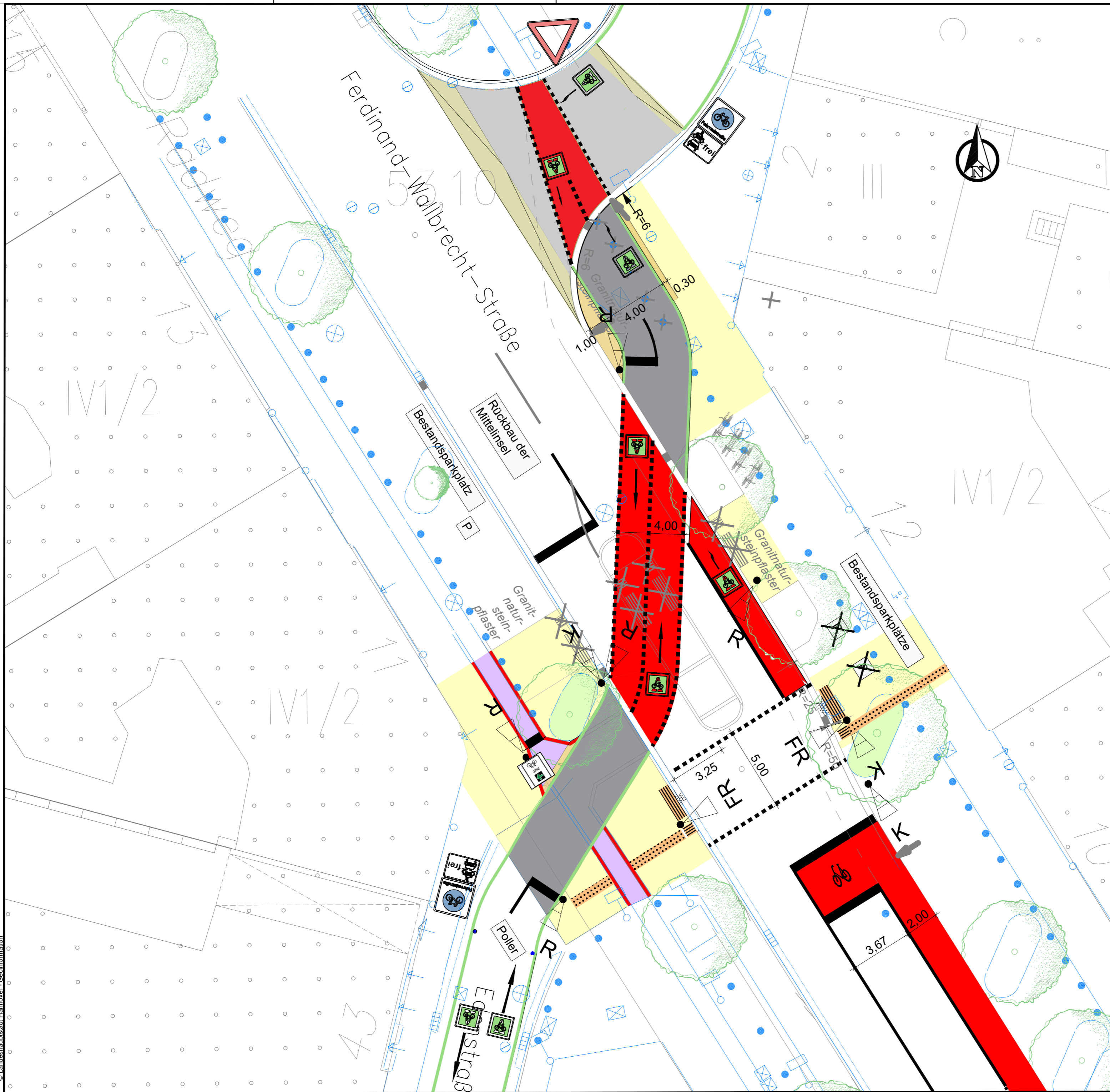
Übersichtsplan, Maßstab 1:2000
