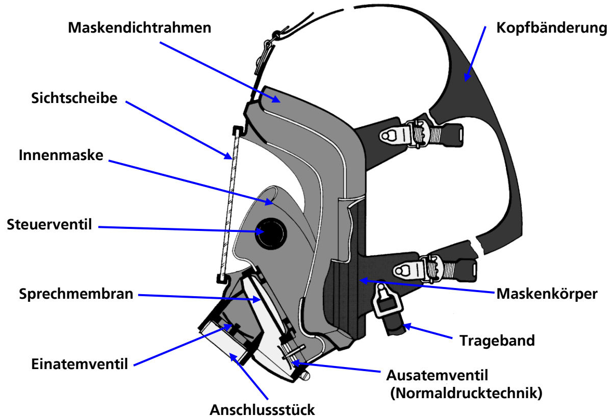
Abbildung 7: Vollmaske (Normaldrucktechnik) Quelle: ursprüngliche Abbildung Dräger (Bearbeitung durch NLBK)
