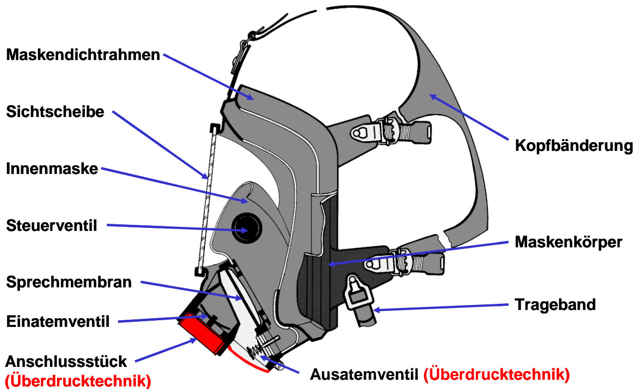
Abbildung 9: Vollmaske (Überdrucktechnik) Quelle: ursprüngliche Abbildung Dräger (Bearbeitung durch NLBK)
