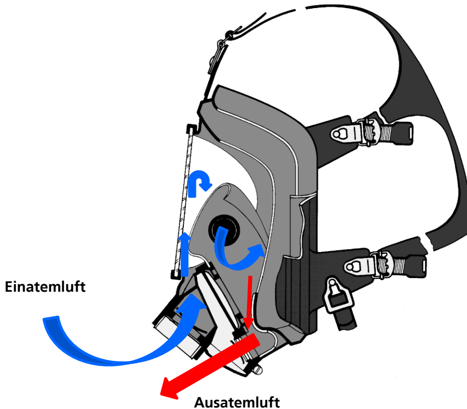
Abbildung 8: Allgemeine Luftführung innerhalb einer Vollmaske Quelle: ursprüngliche Abbildung Dräger (Bearbeitung durch NLBK)
