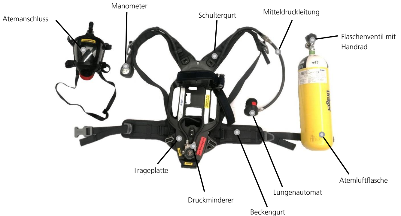
Abbildung 12: Aufbau des Pressluftatmers
